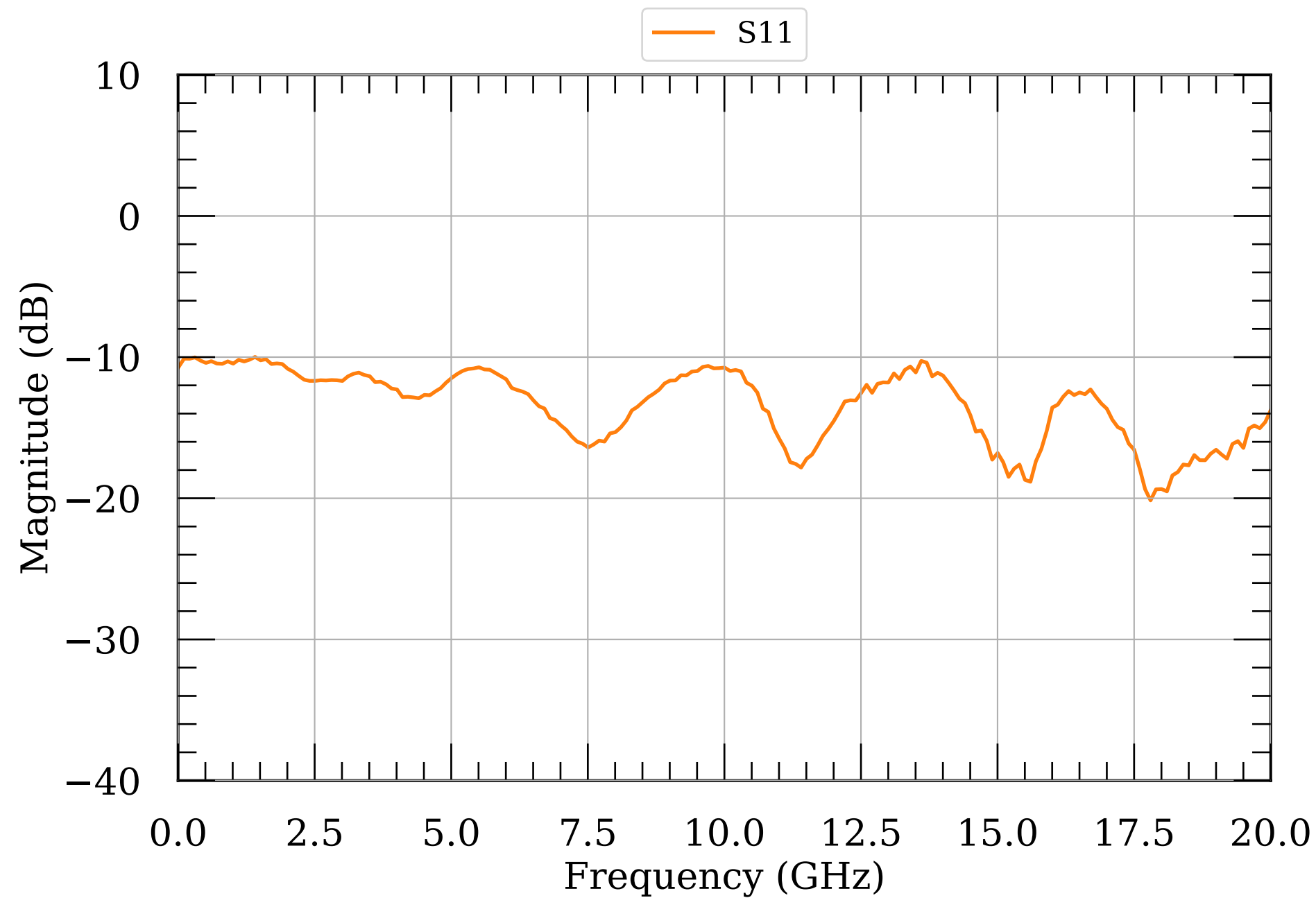
LNA S-params module099
